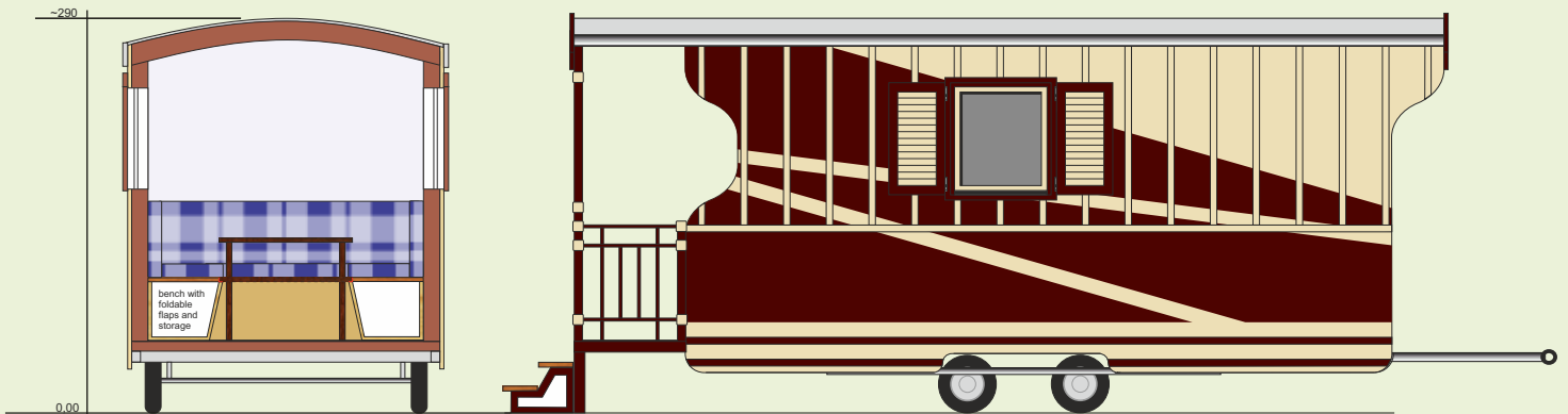
SCHNITT A-A
